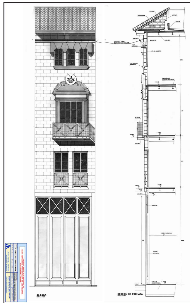
Alzado de la Casa Hermandad. Álvaro Mendiola.
